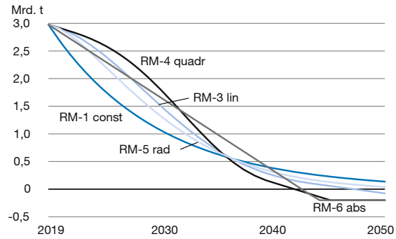
Abbildung 2 Exemplarische EU-Emissionspfade
